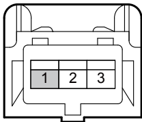
发动机控制模块线束连接器(4G18) EN44
