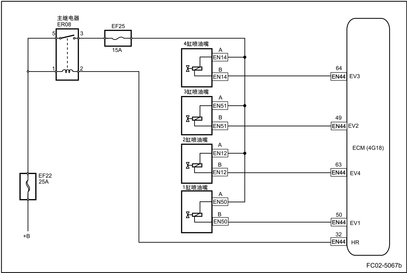
喷油嘴
