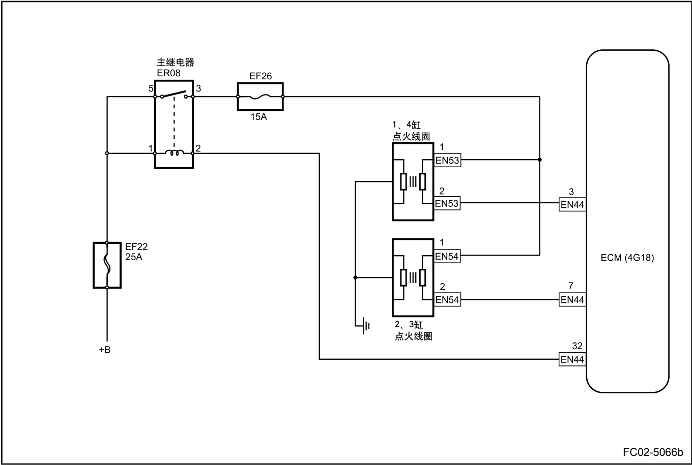
点火系统
