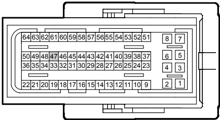
发动机控制模块线束连接器(4G18) EN44
